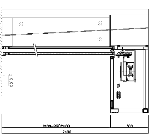
ŘEZ OBLUKOVÉ DVEŘE TRA
